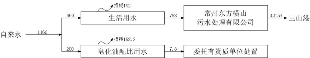
图 2.1-1 水平衡图 单位：m³/a
