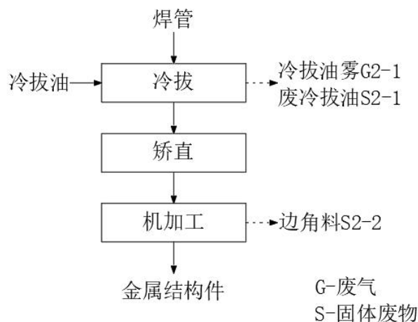
图 2.2-2 金属结构件制造工艺流程及产污环节图
