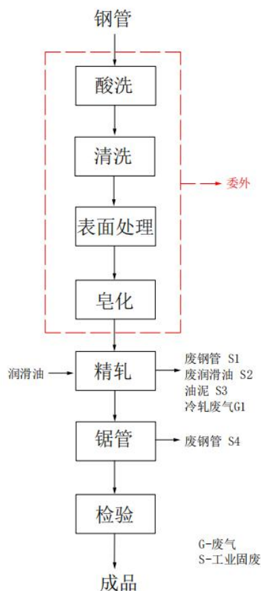
图 2-2 原有项目精密钢管工艺流程图
