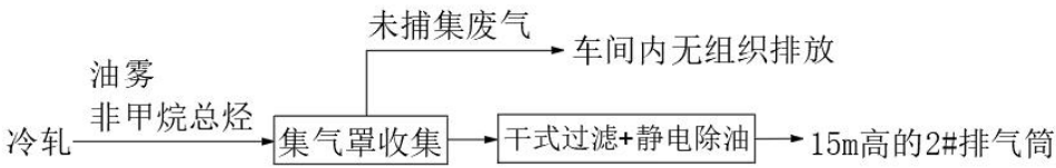
图 4-1 本项目废气处理装置收集方式
