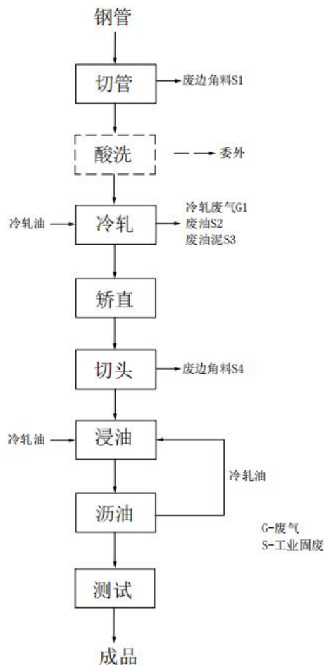
图 2-1 精密钢管制造工艺流程及产污节点图
