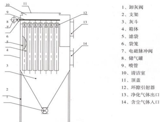
图 4-3 袋式除尘器结构及组成图
