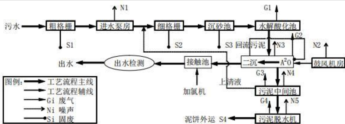
图 4-6 常州东方横山水处理有限公司污水处理工艺流程图
