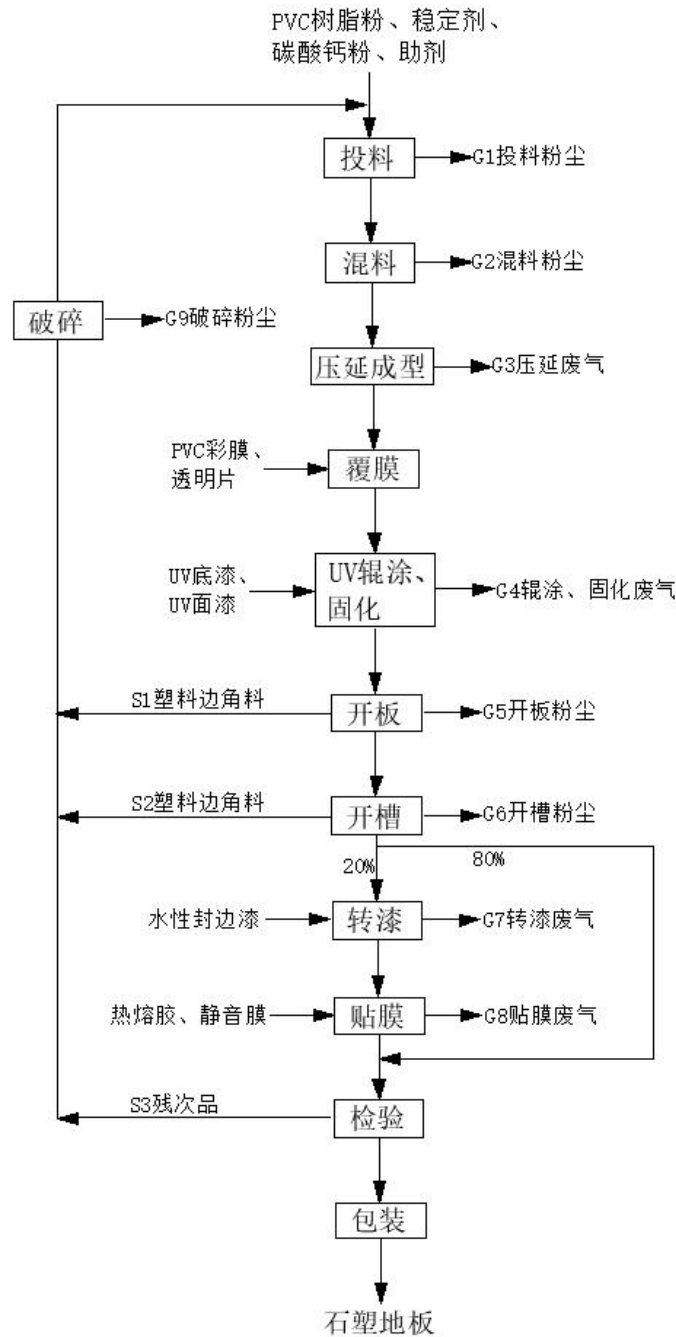
图 2-3 石塑地板生产工艺及产污流程图
