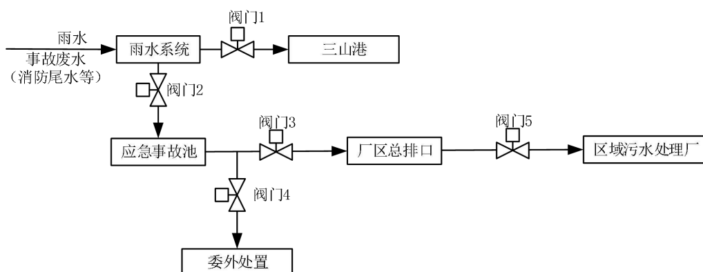
图 4-8 事故排水控制和封堵示意图
