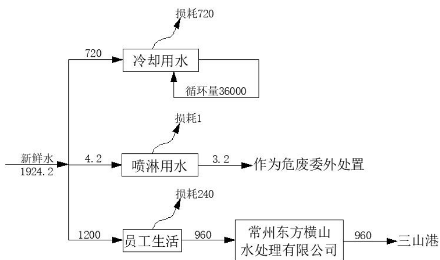
图2-2 本项目水平衡图 (t/a)
