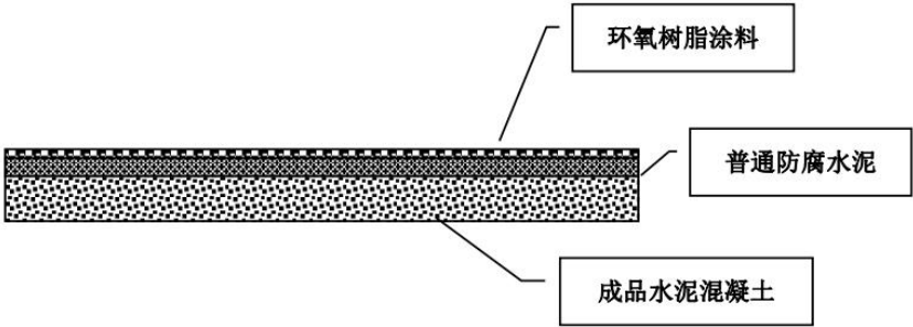
图 4-7 重点防渗区域剖面图
