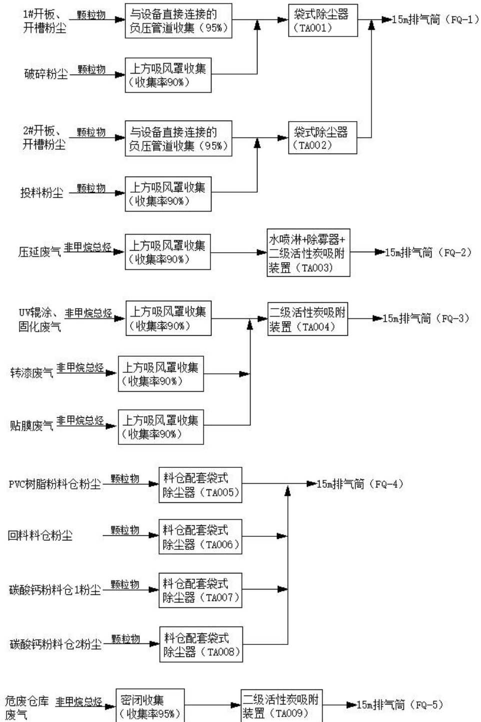
图 4-1 本项目废气收集处理示意图
