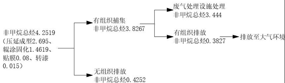
图 2-1 非甲烷总烃平衡图 (t/a)
