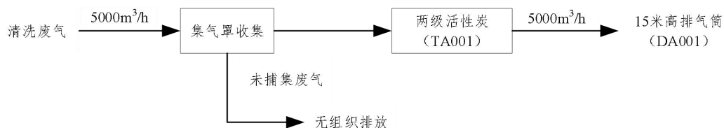
图 4-1 企业废气处理工艺图
