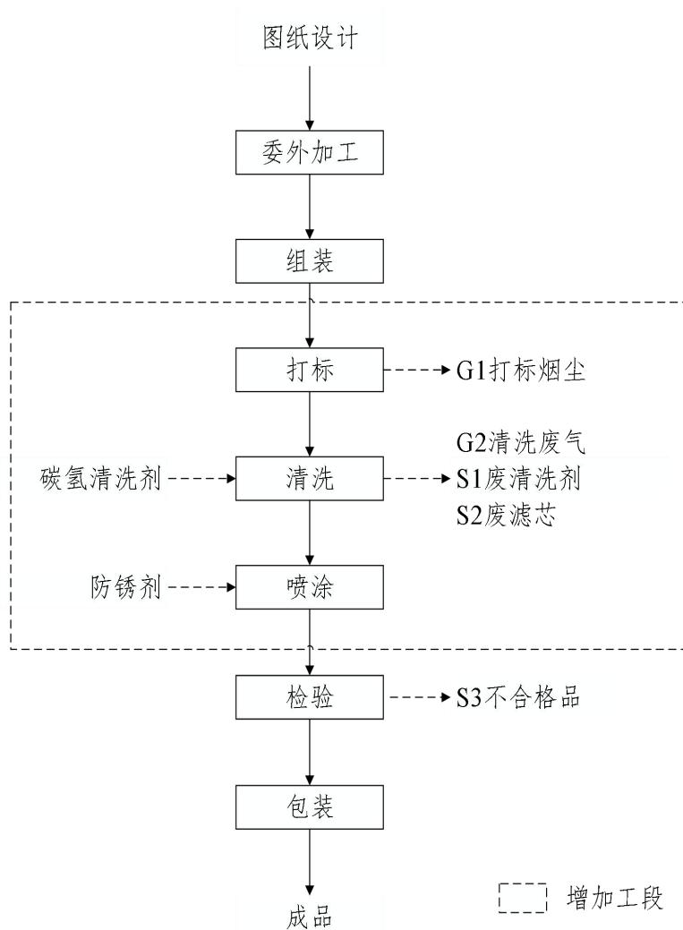
图2-3 工艺流程图
