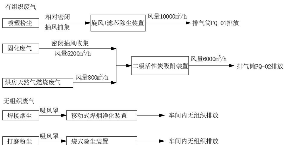
图 4-1 本项目废气收集处理流程图
