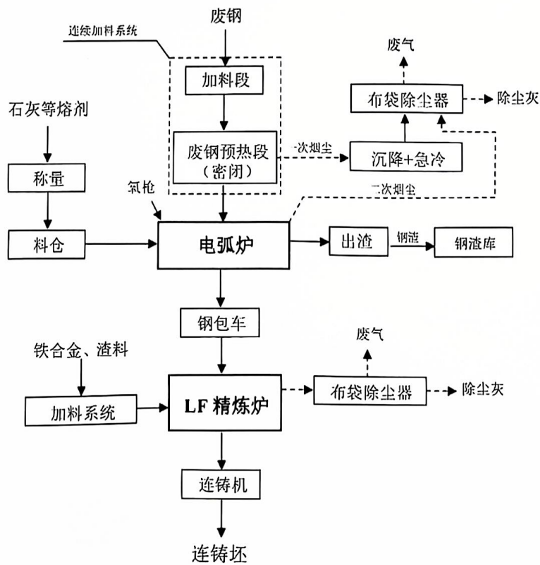
图 3.1.3.3 现有项目电炉-精炼工艺流程图
