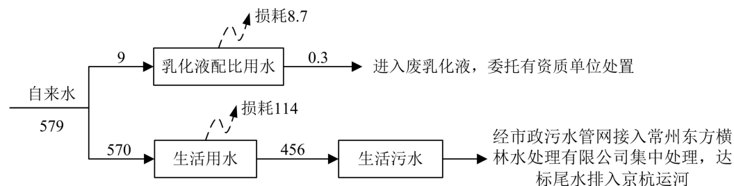
图 2-3 本项目水平衡图（单位：t/a）
