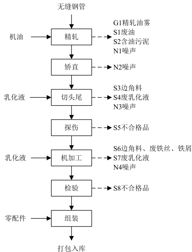
图 2-5 生产工艺流程图
