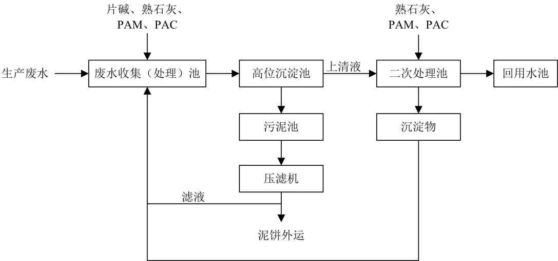
图 2-7 生产废水处理工艺流程图
