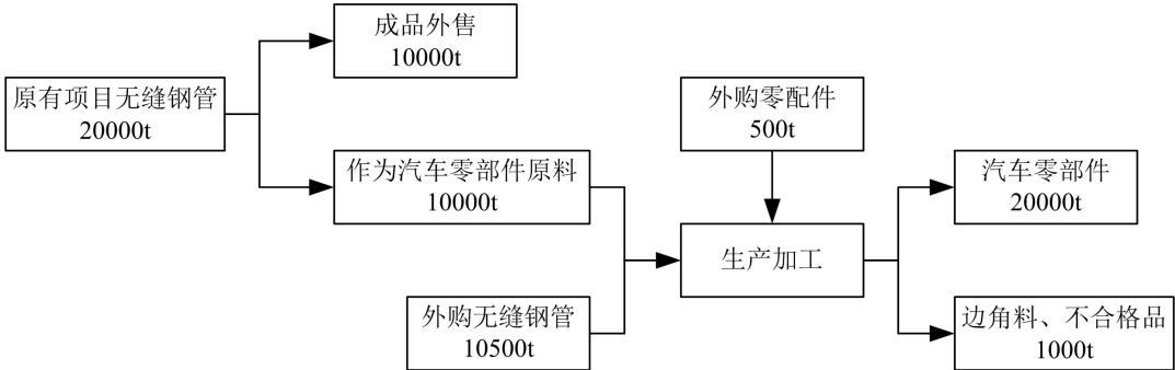
附图 2-1 产品流向图
