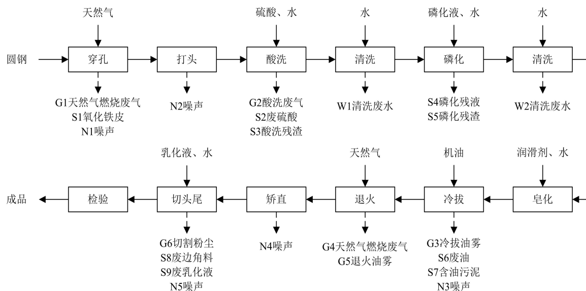
图 2-6 原有项目生产工艺流程图
