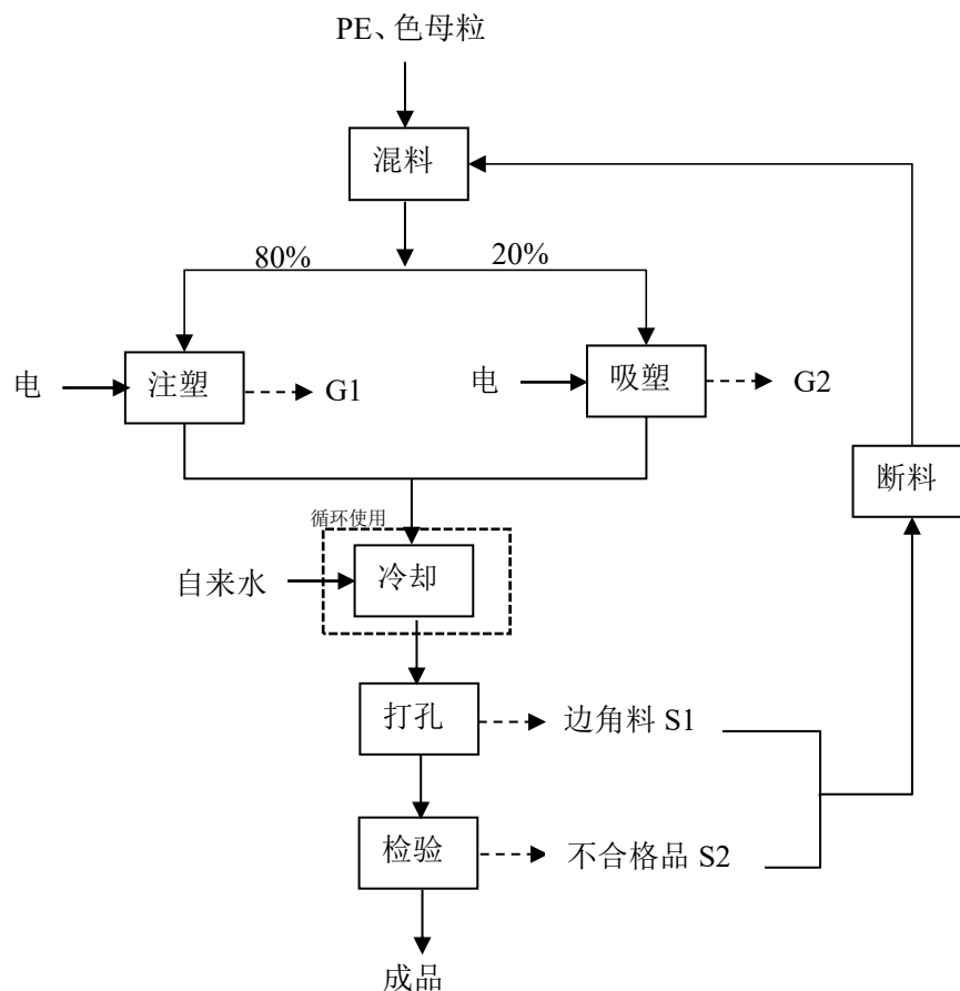
图 2.2-1 汽车保养设备制造工艺流程及产污环节图
