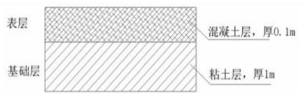
图 4-3 一般防渗区域剖面图
