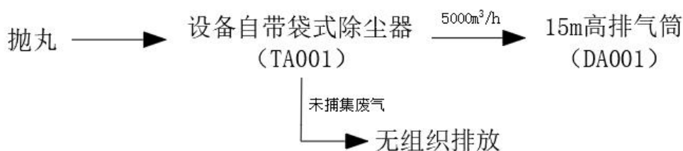
图 4-1 企业废气处理工艺图
