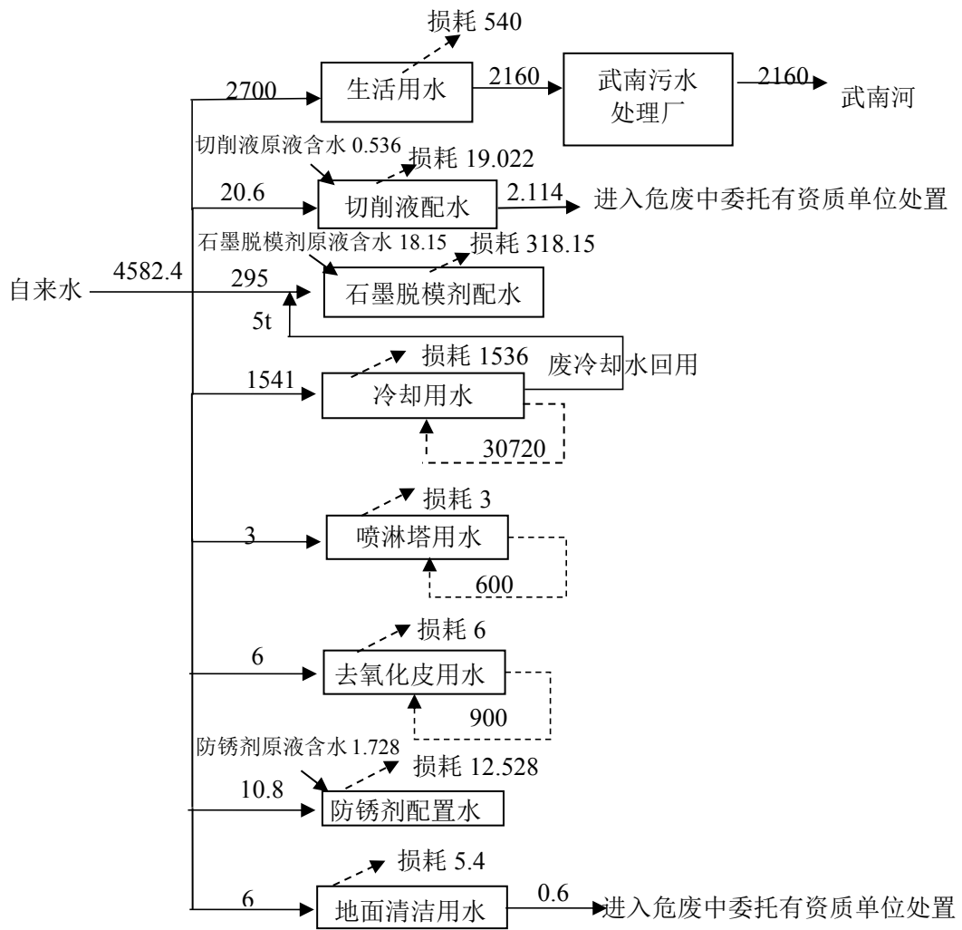
图 2-2 本项目水平衡图 (t/a)
