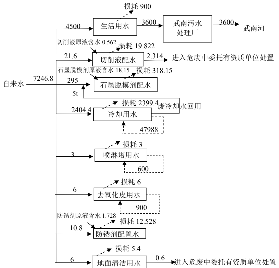
图 2-3 全厂水平衡图 (t/a)
