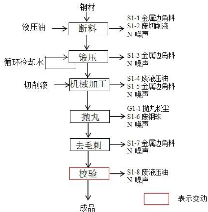
图 2-6 原项目生产工艺流程图
