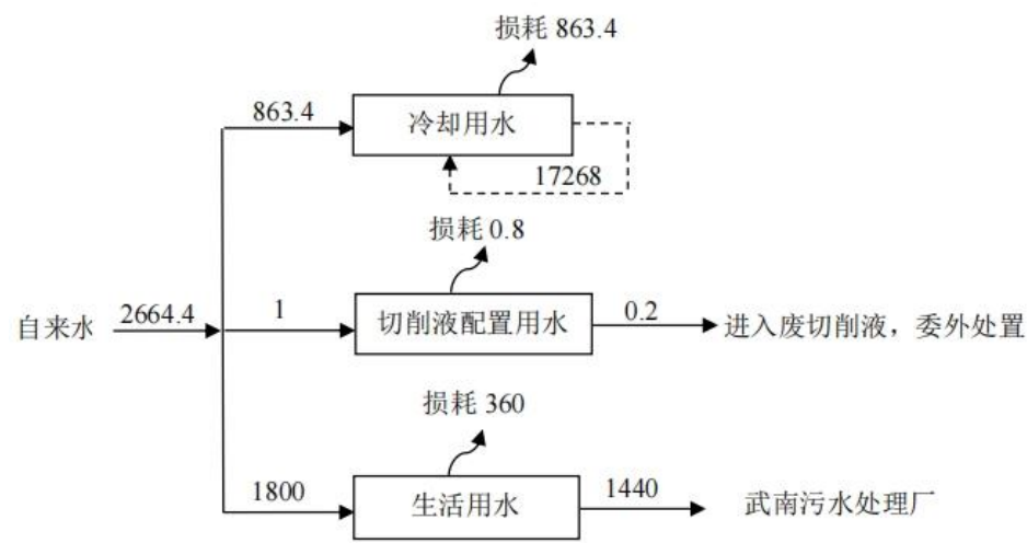
图 2-7 原环评中水平衡图
