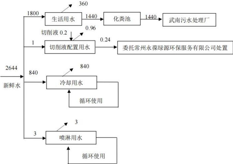
图 2-9 原项目实际水平衡图
