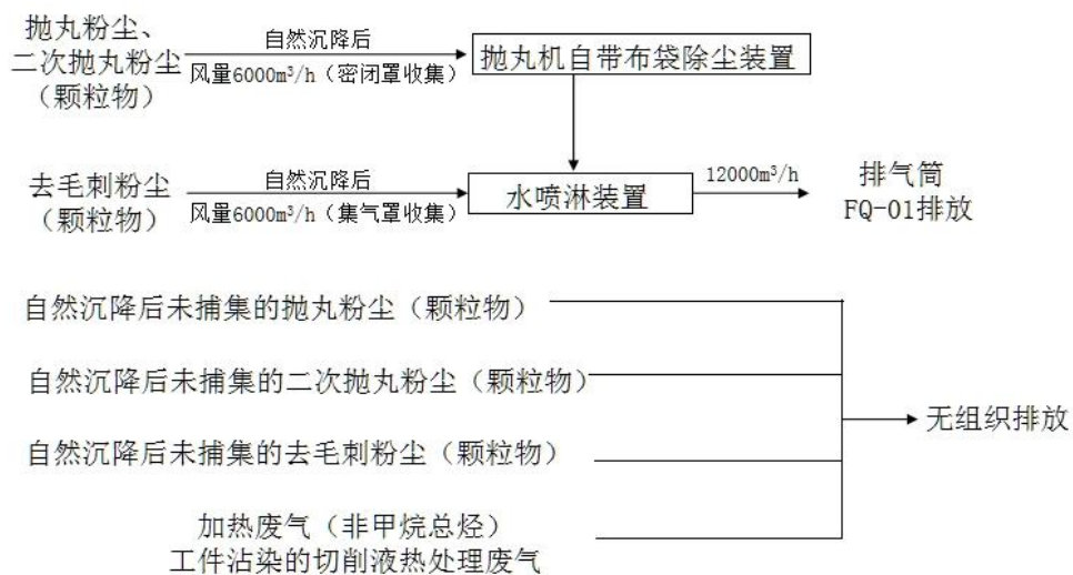
图 4-1 本项目投产后全厂废气收集治理工艺图
