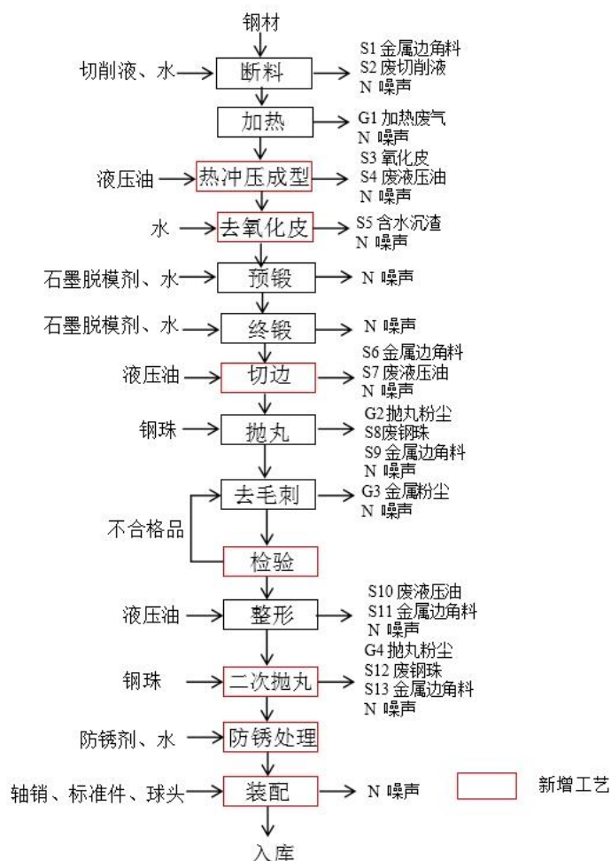
图 2-4 汽车门铰链工艺流程图
