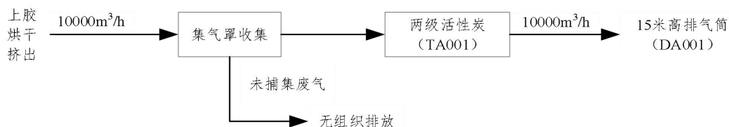
图 4-1 企业废气处理工艺图
