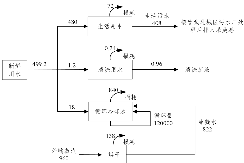
图 2-2 项目水平衡图 (t/a)
