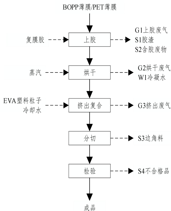
图2-3 工艺流程图
